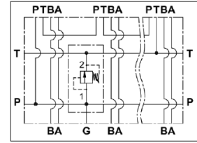
SERIE CIRCUIT WITH OPTIONAL RELIEF VALVE SHOWN
